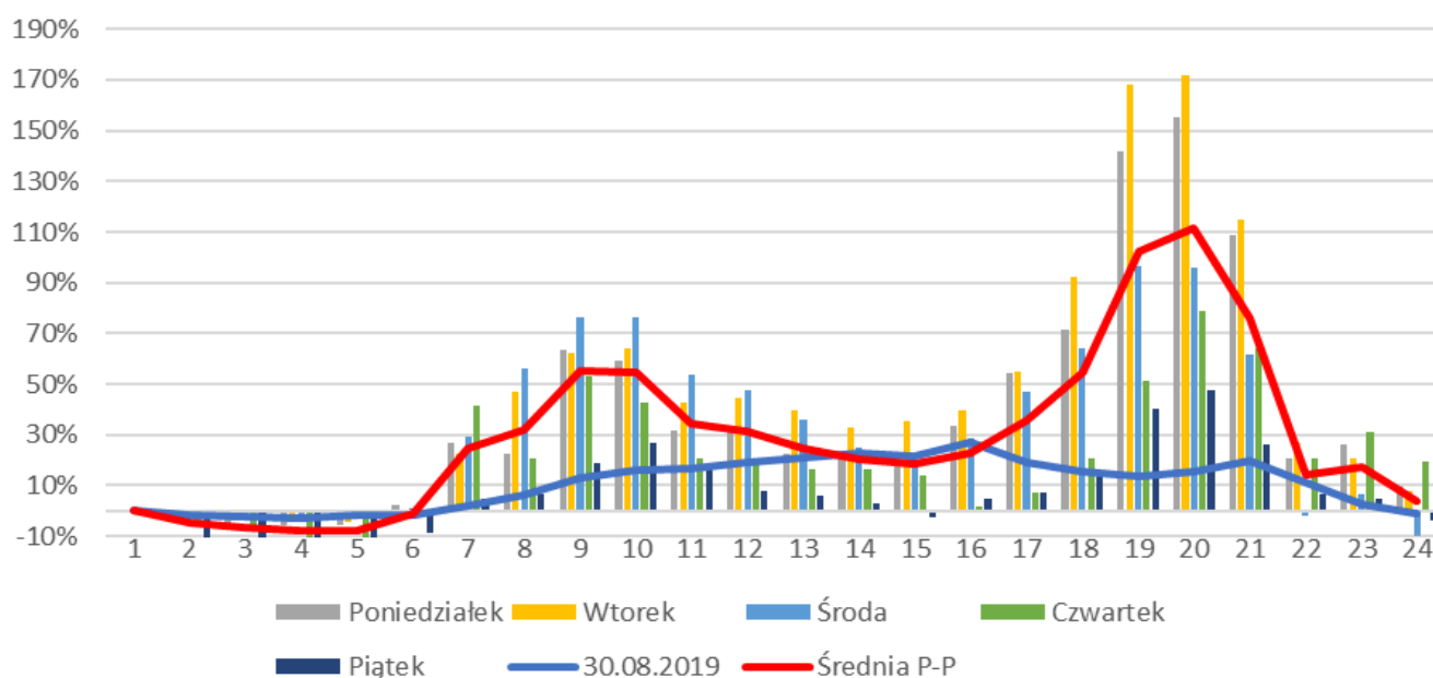
Dynamika zmian cen godzinowych energii elektrycznej - RDN - dni robocze 11.10 - 15.10.2021 r. - godzina 0-1 baza
